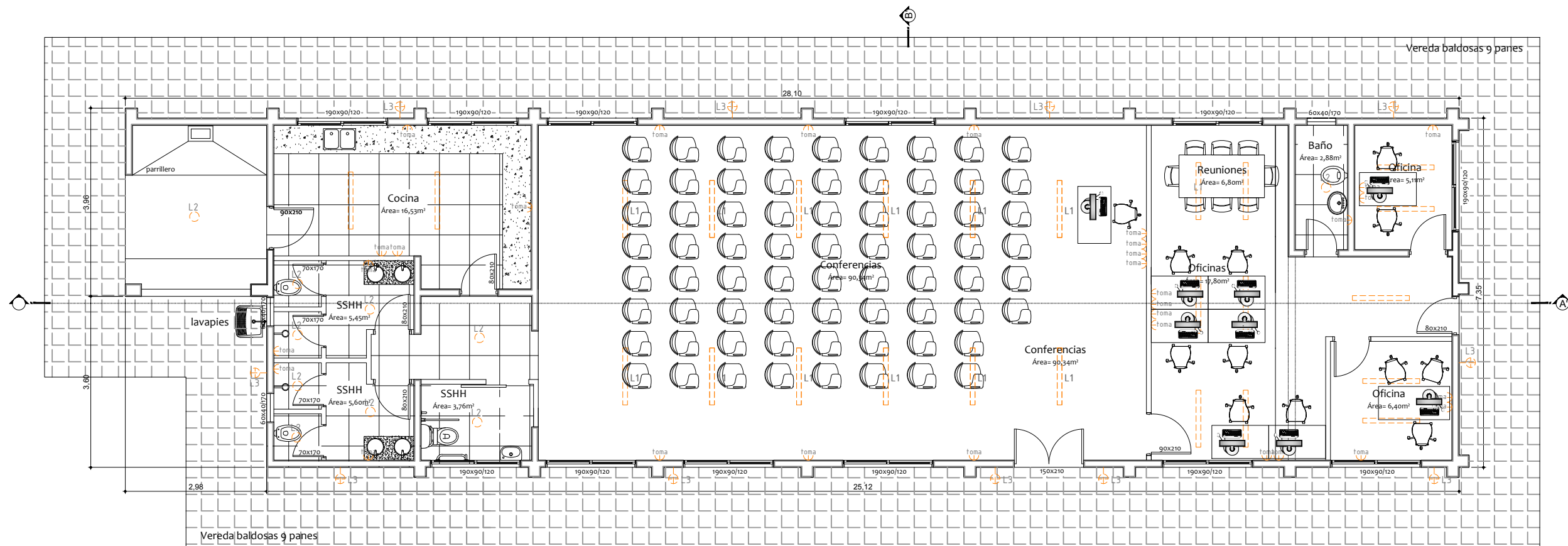
Planta baja mobiliario
