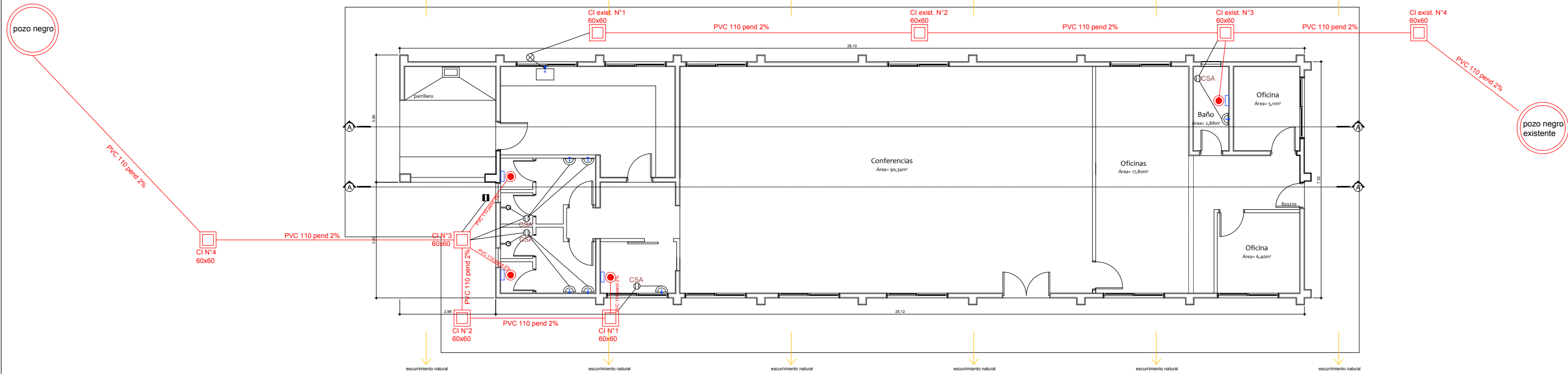
Planta baja sanitaria Esc.: 1/125
