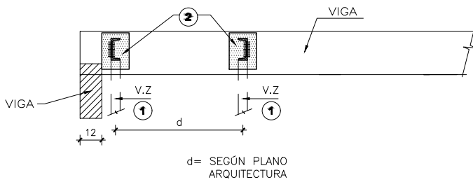
DET 02 APOYO VIGAS ZANCA (V.Z) EN VIGA DE ENTREPISO
