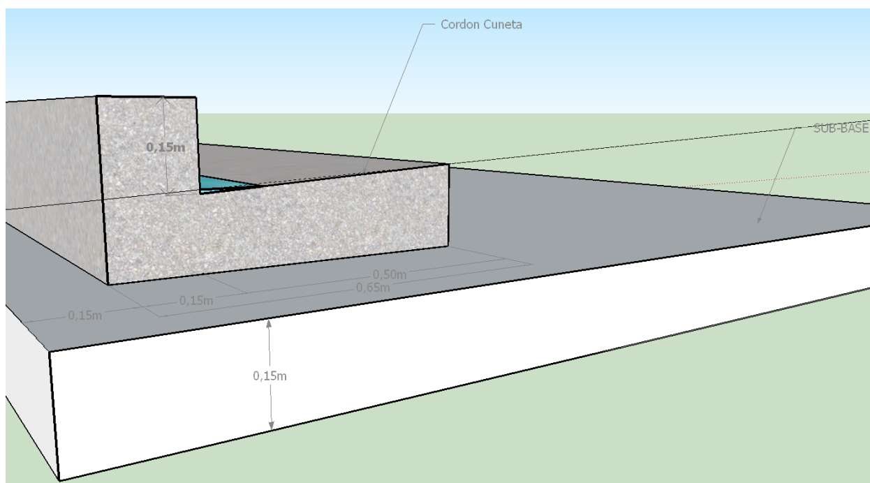
Figura 01: Detalle Típico Cordón Cuneta Sobre Sub-Base
