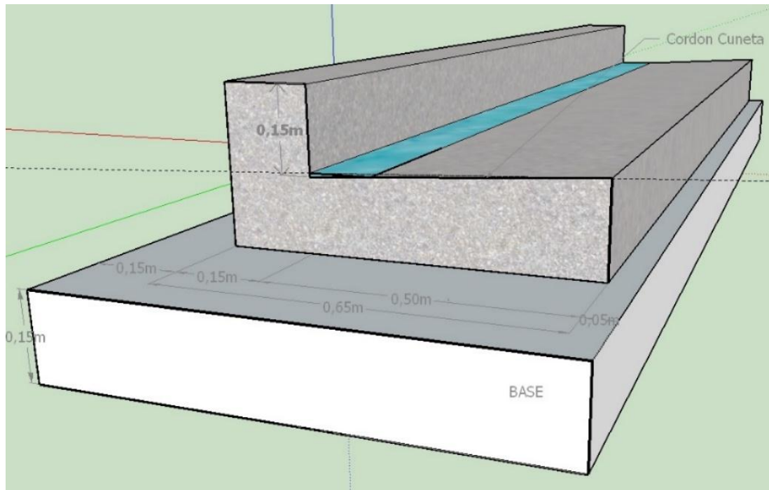
Figura 01: Detalle Típico Cordón Cuneta Sobre Base granular
