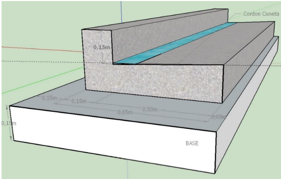
Figura 01: Detalle Típico Cordón Cuneta Sobre Sub Base granular
