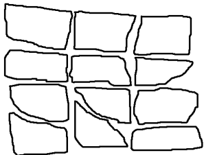
Junta corrida (incorrecto)
