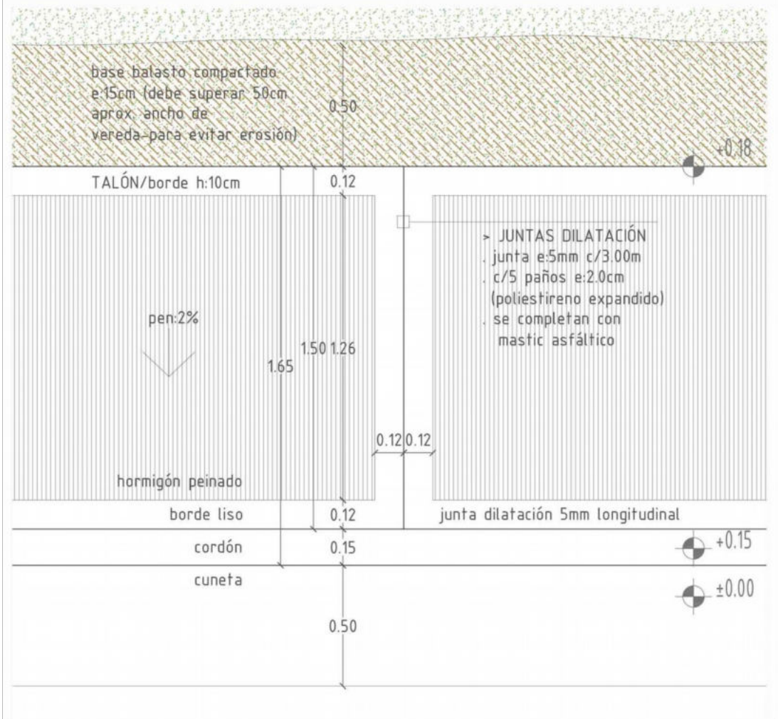
Detalle Vereda 1.50m Planta - esc:1/20
