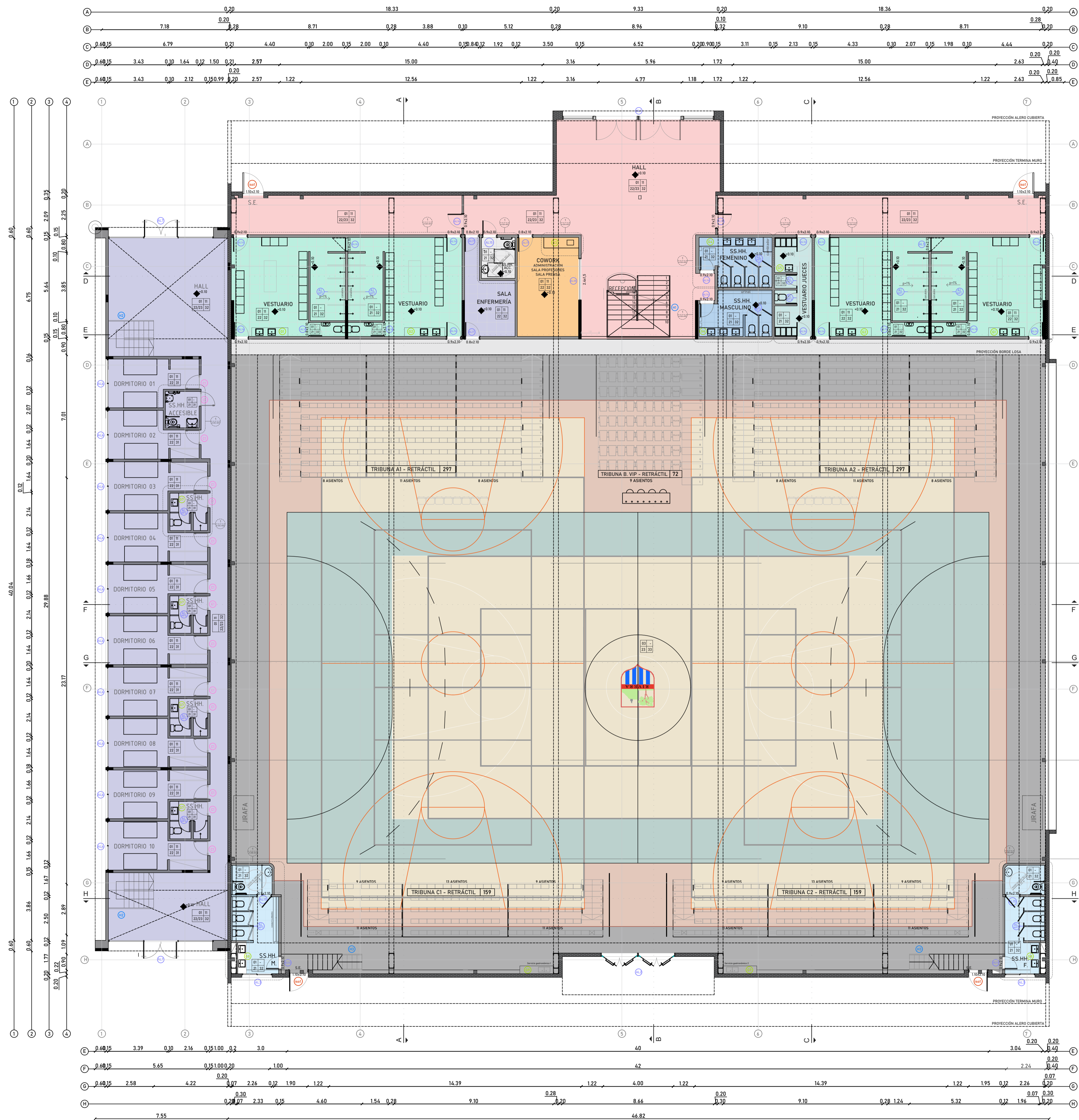
PLANTA BAJA escala 1:120
