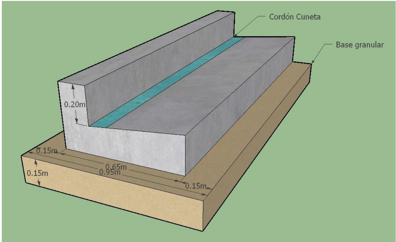
Figura 01: Detalle Típico Cordón Cuneta Sobre Base granular
