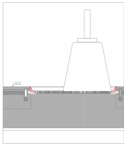
Le4 perfil LED embutido en borde
