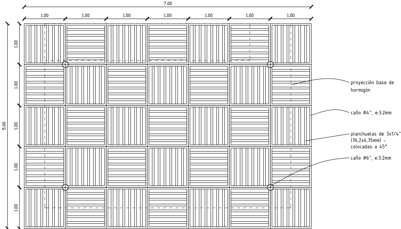
PLANTA BAJA PÉRGOLA METÁLICA | esc. 1/50
