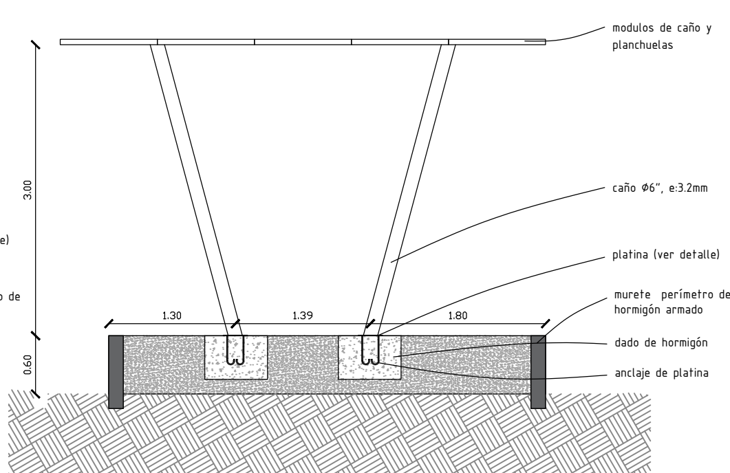
CORTE TRANSVERSAL | esc. 1/50
