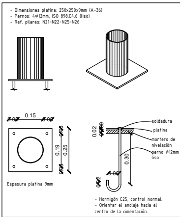
DETALLE PLATINA | esc. 1/20
