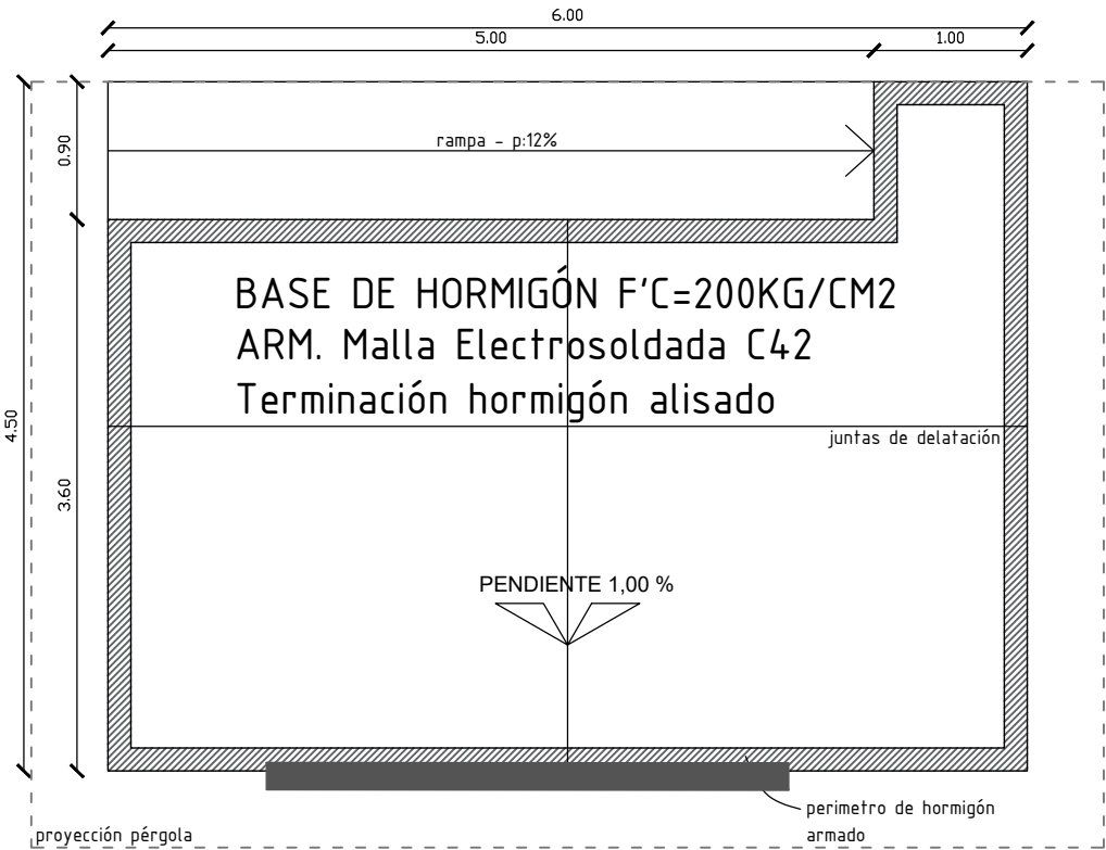
PLANTA BAJA BASE DE HORMIGÓN | esc. 1/50
